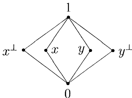
Fig. 1. Lattice MO2.
